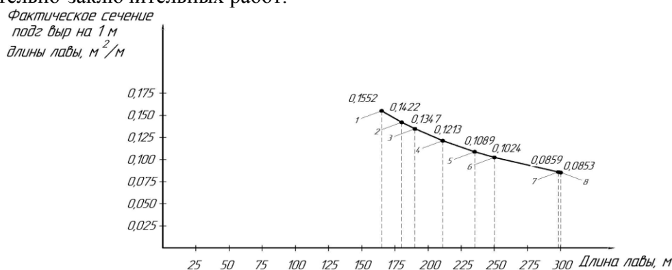
Рис.4. График зависимости удельного сечения подготовительных выработок в свету на 1 м длины очистного забоя от длины лавы
