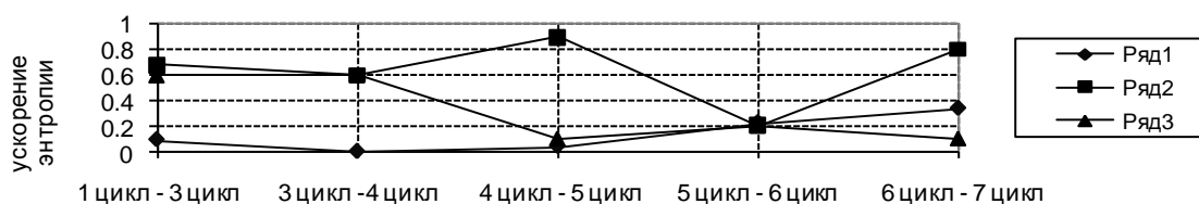
Рис. 3.а. Зависимость ускорения энтропии песчаника (шх. им. Ленина, гор. 800 м, "кубик") от числа циклов нагружения при различных температурах: 1 - 20 0 С; 2 - 30 0 С; 3 - 50 0 С.
